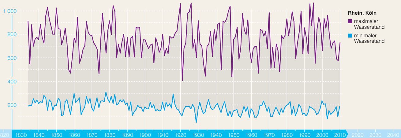
▶ Abb 3 Maximale und minimale Wasserstände — in cm
