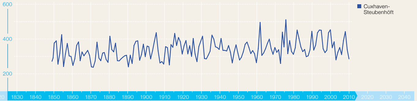
▶ Abb 4 a Höchste Wasserstände Nordsee — in cm, höchster Wert des Tidehochwassers (HThw)
