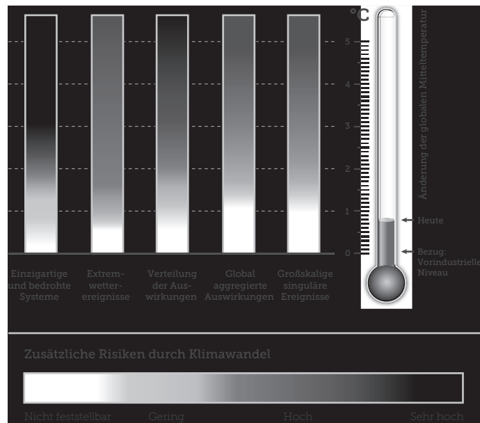
Abb. 1: Anstieg der globalen Mitteltemperatur und die damit verbundenen Risiken. Quelle: IPCC (2014a)
