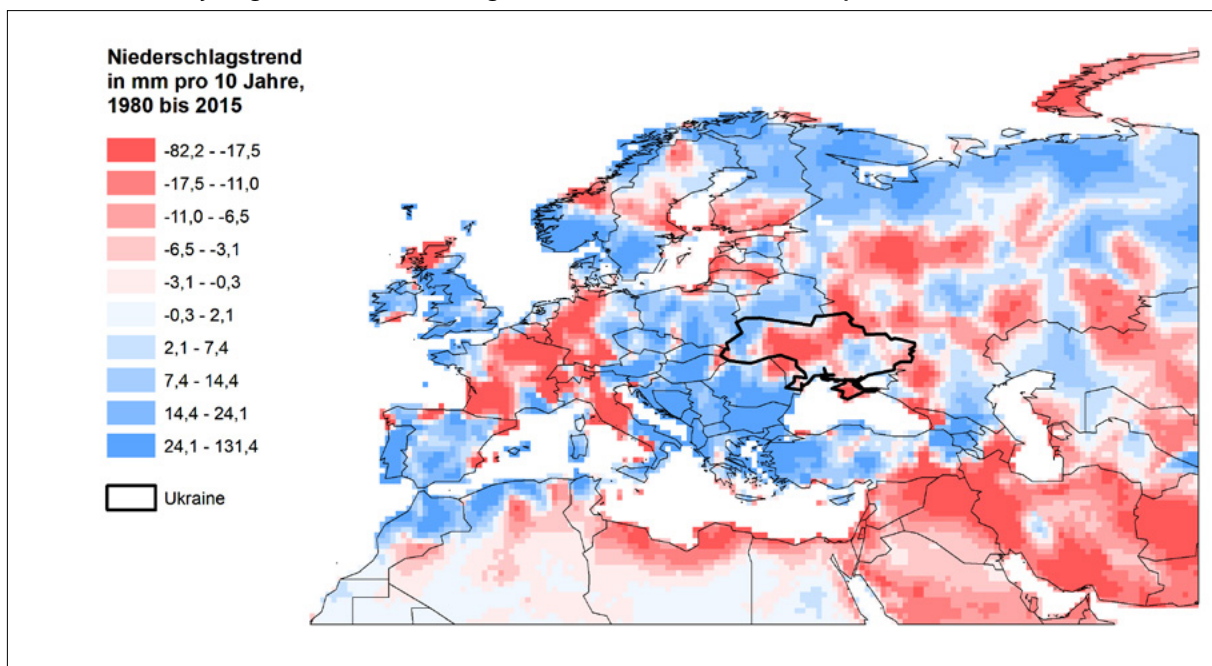
Grafik 2: Ganzjährige, lineare Niederschlagstrends von 1980 bis 2015 in Europa
