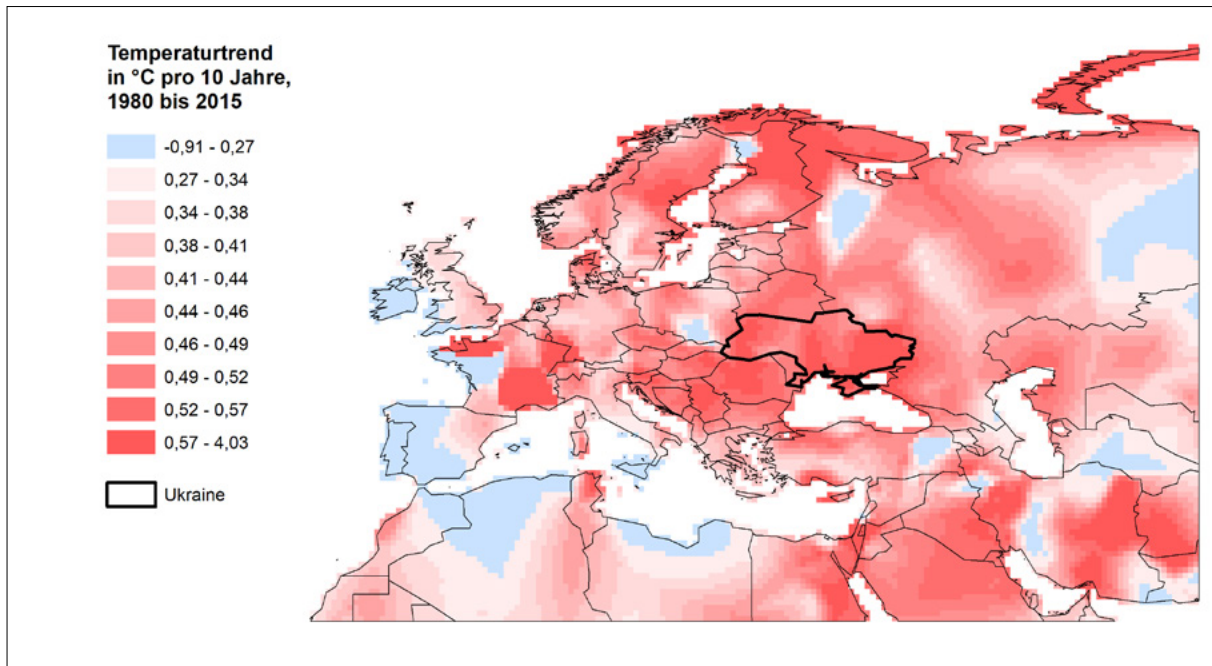
Grafik 1: Ganzjährige, lineare Temperaturtrends von 1980 bis 2015 in Europa
